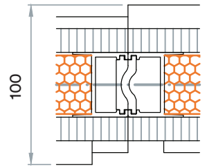
nodo con profili nascosti knot detail of hidden profiles
